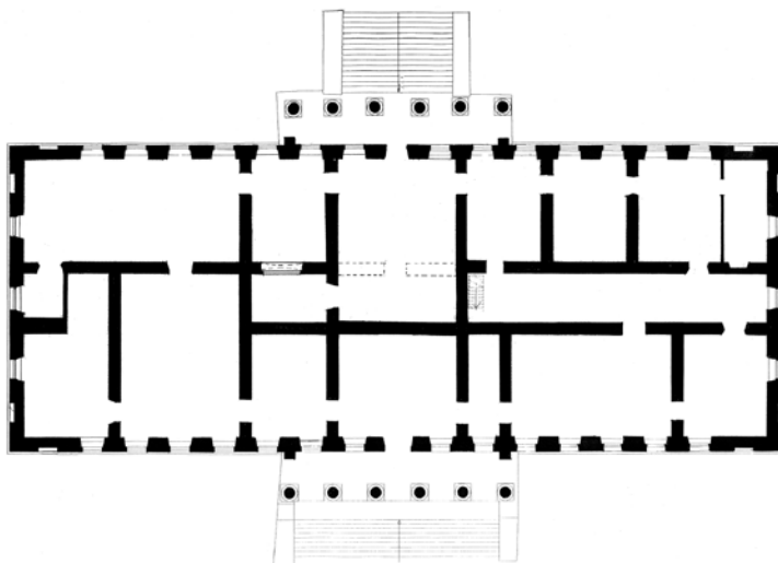
11. Arnionių rūmų XVIII a. pab. plano rekonstrukcija, pagal R. Zilinsko brėžinį ir tyrimus braižė Sigita Kynienė, 2016
